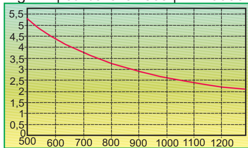
Fig. 77 | curbare la rece | R = 6000 mm
