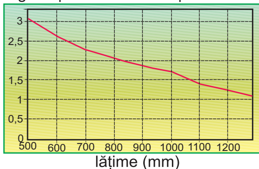
Fig. 35 | curbare la rece | R = 3000 \text{ mm}
