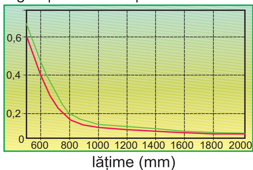
Fig. 6 | curbare la rece | R = 667 \text{ mm}
