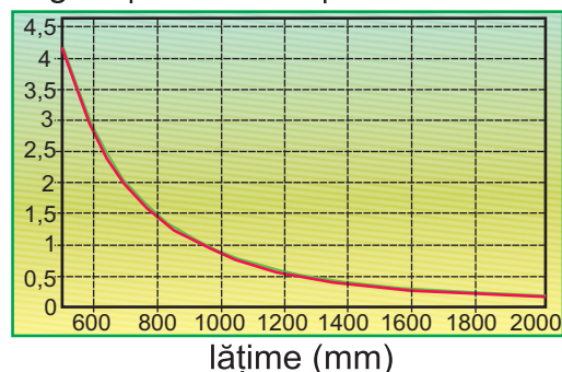
Fig. 58 | curbare la rece | R = 4000 \text{ mm}
