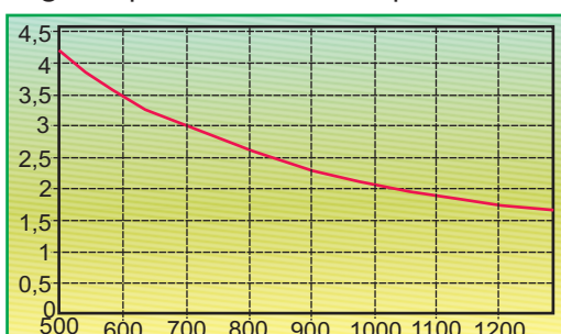
Fig. 78 | curbare la rece | R = 7000 mm
