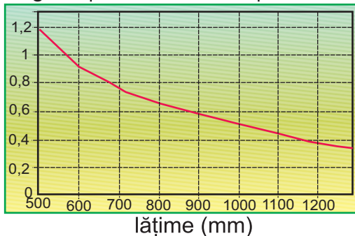
Fig. 18 | curbare la rece | R = 2500 \text{ mm}
