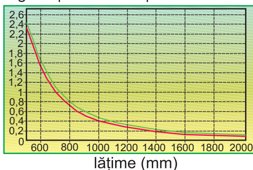
Fig. 33 | curbare la rece | R = 1667 \text{ mm}
