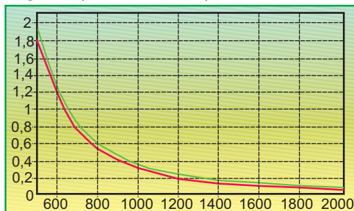
Fig. 22 | 4 reazăme | L = 2000 mm
