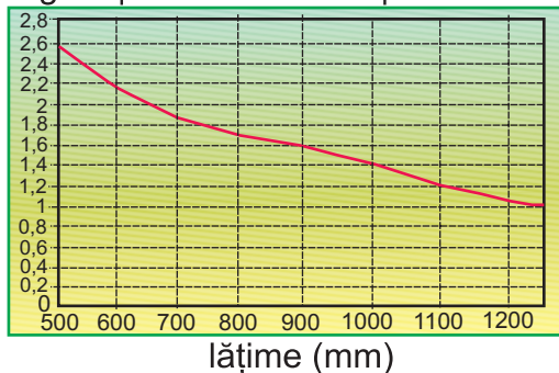
Fig. 17 | curbare la rece | R = 2000 \text{ mm}
