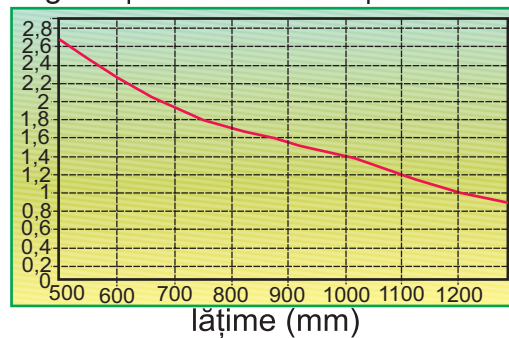
Fig. 36 | curbare la rece | R = 3500 \text{ mm}
