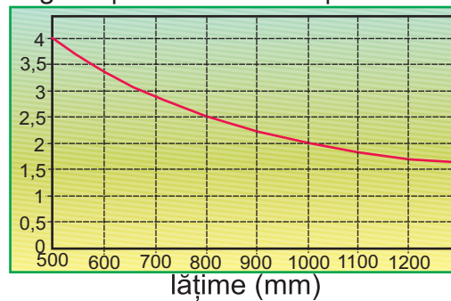
Fig. 69 | curbare la rece | R = 6000 mm
