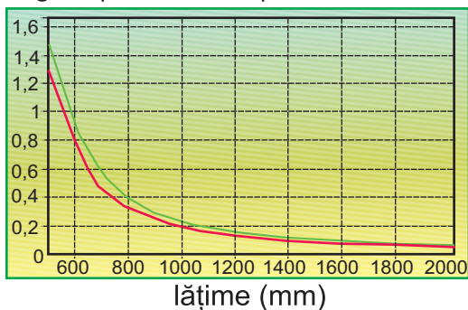
Fig. 15| curbare la rece | R = 1000 \text{ mm}
